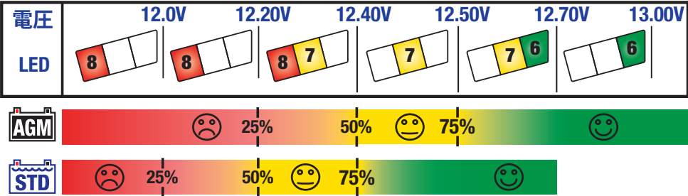
SOH健康診断テスト結果:12V鉛電池(プログラム 1 & 2)
