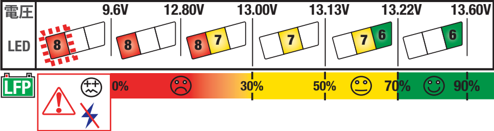
SOH健康診断テスト結果:リン酸鉄リチウム電池(プログラム 3 & 4)
